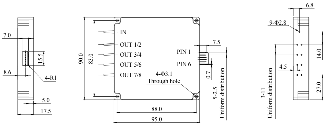
图 1. 外观尺寸
