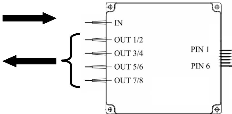
图 2. 产品工作在 1×8 光开关方式
